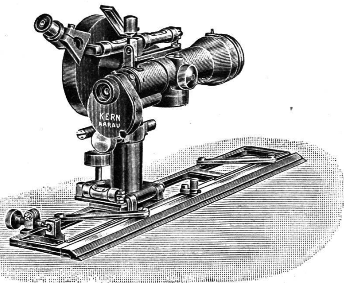
Kippregel Nr. 79
