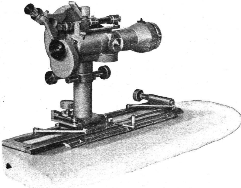
Kippregel Nr. 79
