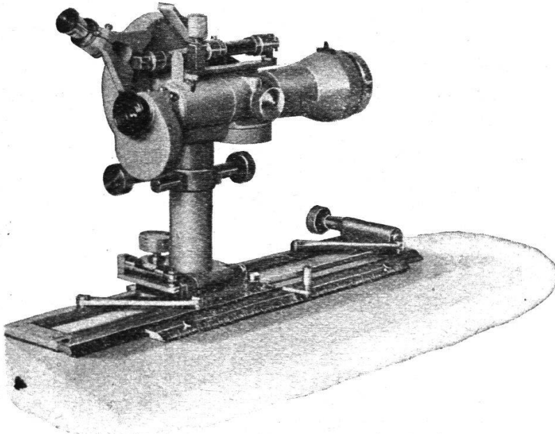
Kippregel Nr. 79
