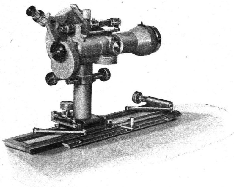
Kippregel Nr. 79
