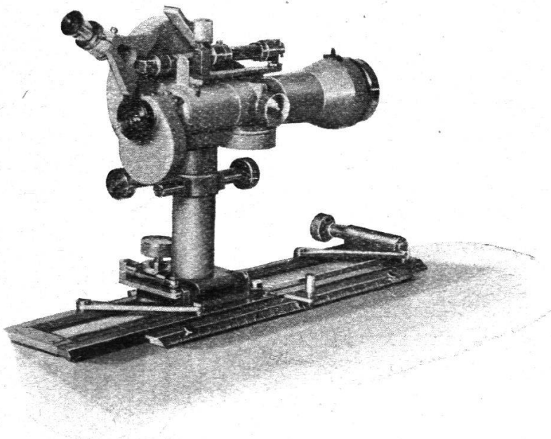
Kippregel Nr. 79
