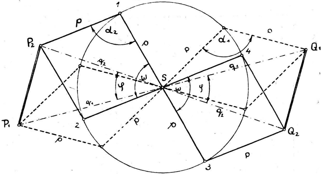
Abb. 1. Nürnberger-Schere
