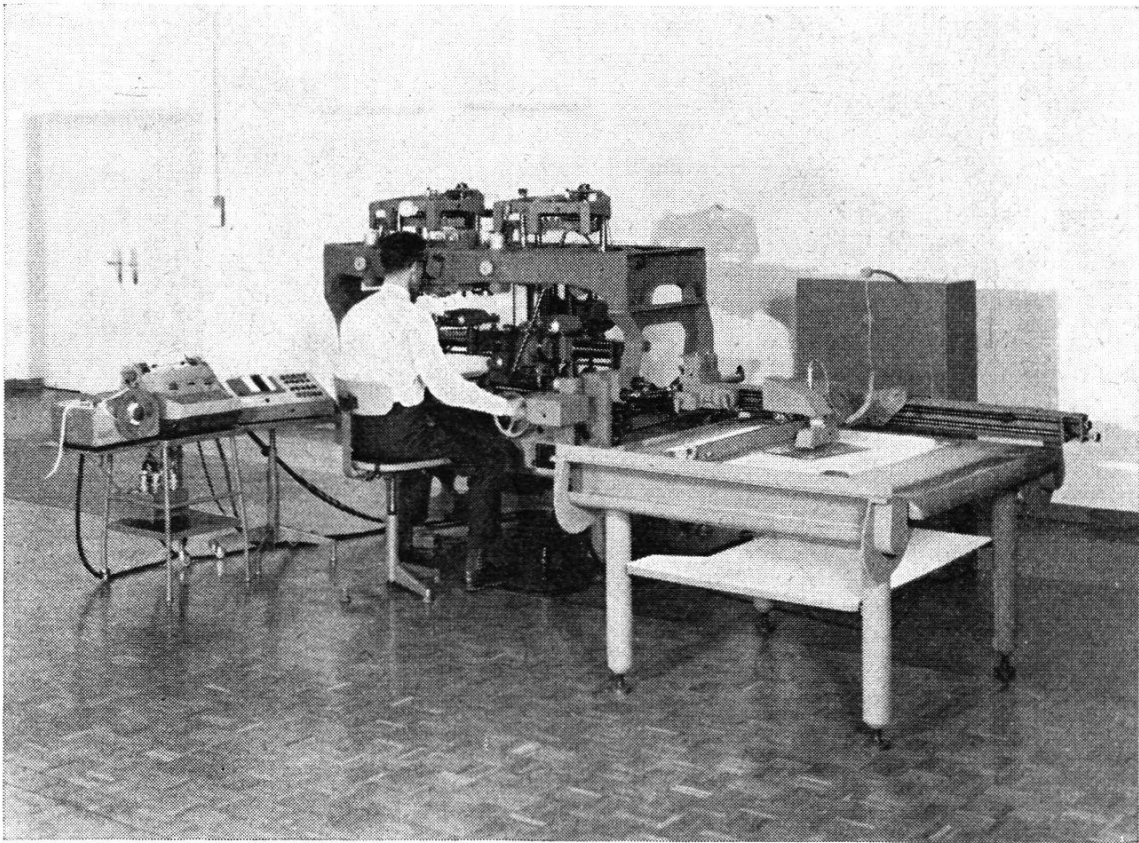
Universal-Stereoautograph Wild A 7 mit Zeichentisch, elektrischem Koordinaten-Registriergerät Wild EK 5 und Streifenlocher Wild SL 15. Die Anlage gestattet, das Modell des Geländes in der Form des Stereoluftbildes im Zimmer wiederzugeben und daran jede Art graphischer oder zahlenmäßiger Geländevermessung auszuführen
