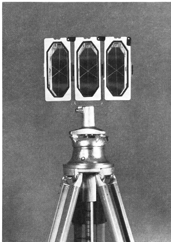
Abb. 7 Drei mit Bajonettverschlüssen zusammengekuppelte Reflektoren auf einem Zentrierstativ.
