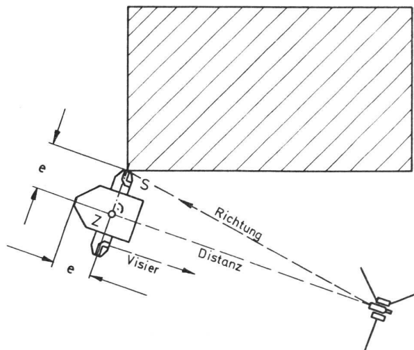
Abb. 4 Z Zentrum in der Kippachse des Reflektors; e feste bekannte Exzentrizitäten; S einsteckbare Zapfen in der Kippachse des Reflektors mit Winkelvisier.
