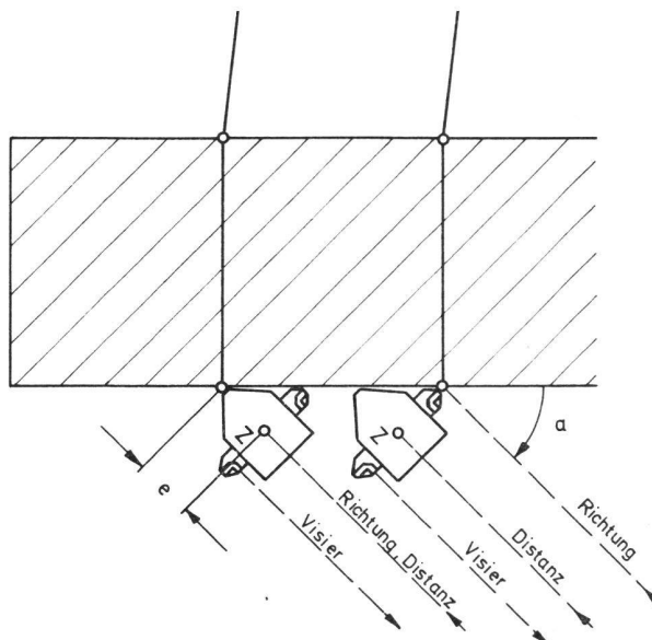
Abb. 5 Grenzfälle: Links wird die Distanz um e zu klein gemessen, hingegen braucht für die Richtungsmessung nicht neu gezielt zu werden. Rechts wird die gleiche Aufnahmesituation so behandelt, wie in Abb. 4 dargestellt ist.
