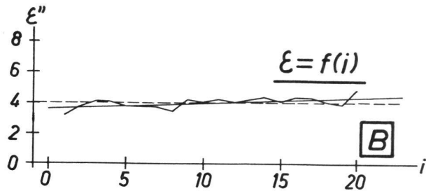
Abb. 3 Versuch B. Meßreihe mit dem NA 2 am 3. Februar 1972. i : Laufende Nummer der Messung. \varepsilon : Neigung der Zielachse. Gestrichelt: mittlere Zielachsenneigung. Ausgezogene Gerade: ausgleichende Gerade (Regressionsgerade)
