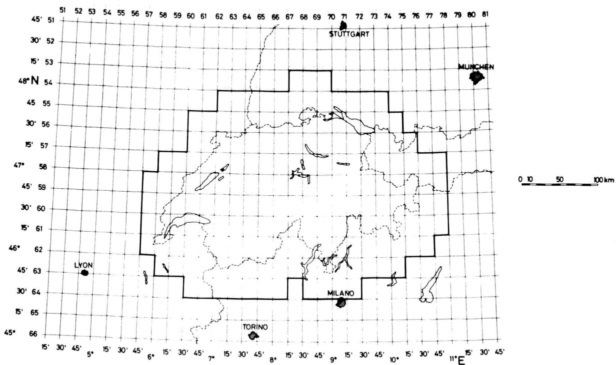
Abbildung 4 Topographische Modelle (A) Modell für die Bestimmung der Geländewirkung im Entfernungsbereich 2,5 \text{ km} \leq r_j \leq 26 \text{ km} Grösse der Rastereinheit: 1' \times 1' In den dargestellten Rechtecken sind 15 \times 15 Einheiten zusammengefasst
