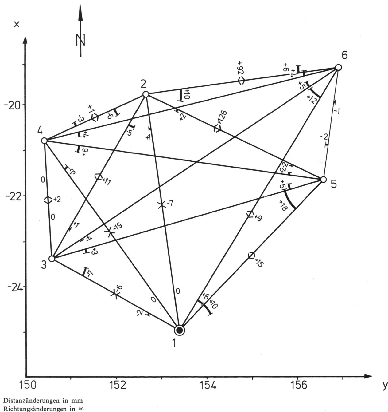
Abb. 5 Einflüsse der Modellfehler der konventionellen Ausgleichung auf die Messgrößen.
