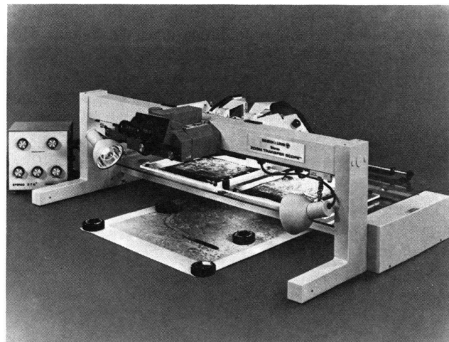
Abb. 2 Luftbildumzeichngerät mit stereoskopischer Betrachtung. (Stereo Zoom Transferscope Bausch & Lomb.)
