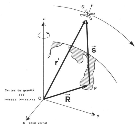
Fig. 10 La relation vectorielle fondamentale liant le centre de gravité des masses terrestres, la station P et le satellite S
