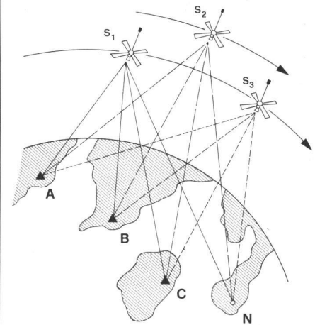
Fig. 7 Principe de la trilatération spatiale
