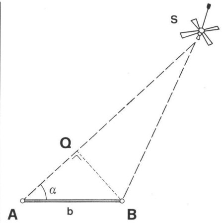
Fig. 6 Détermination électronique d'une direction par le principe de l'interférométrie
