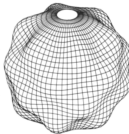
Fig. 11 Représentation de la fonction sphérique correspondant au terme P_6^0 de l'équation (5)
