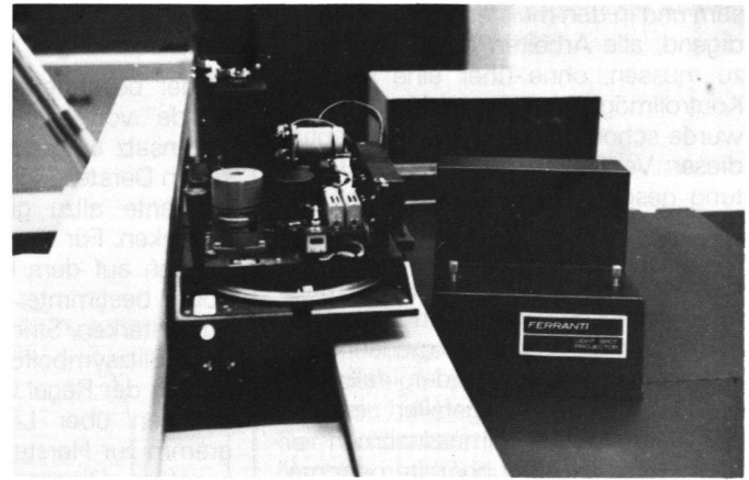
Abb. 2 Lichtzeichenkopf
