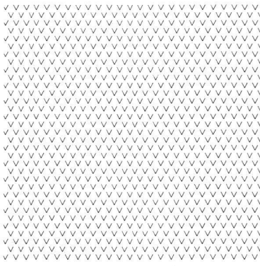
M 10: H = 8%, K = 0,33 S 6 Ostalpin und Südalpin
