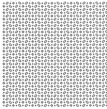
M 3B: H = 15%, K = 0,44 S 8 Tertiäre Intrusionen
