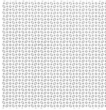
M 3A: H = 12%, K = 0,44 S 8 Tertiäre Intrusionen
