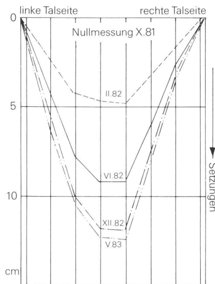
Abb. 5 Schnitt B-B parallel zur Dammachse. Setzungen der Oberflächenpunkte.
