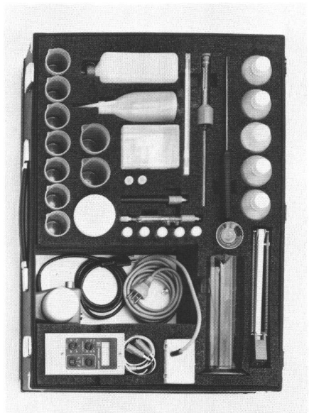
Abb. 1 Einblick in den 68x47x19 cm grossen Analytikoffen des InFieldlabors für chemische Bodenanalysen. In der Mitte erkennt man die Nitrtelektrode.
