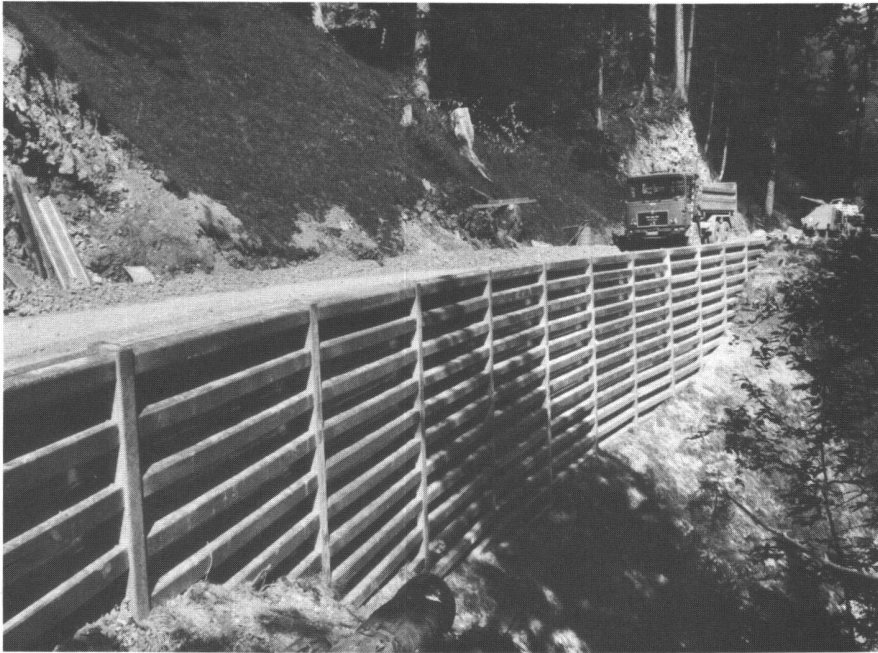
Abb. 3 und 4: Gemeinde Frutigen, Weg Linter. Kassettensstützwände sind praktisch und bewährt, aber wenig landschaftsfreundlich.
