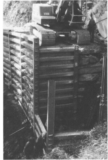
Abb. 3 und 4: Gemeinde Frutigen, Weg Linter. Kassettensstützwände sind praktisch und bewährt, aber wenig landschaftsfreundlich.
