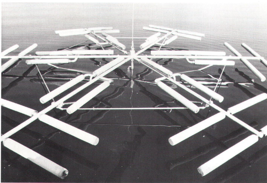
Abb. 3: Das Bild zeigt einen sogenannten Sauerstoffdiffusor. Mit Hilfe dieser Diffusoren werden allen drei Seen (Baldegger-, Hallwiler- und Sempachersee) im Sommer reiner Sauerstoff zugeführt. Pro See sind sechs bis acht solche Einheiten installiert. Im Winter wird das Seewasser mit Druckluft aus Kompressoren durchmischt. Somit ist es möglich, den See mit Sauerstoff aus der Atmosphäre anzureichern.
