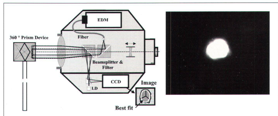
Fig. 1: Image numérique d'un prisme GRZ4 perçue par le capteur CCD d'un TCA1800.
