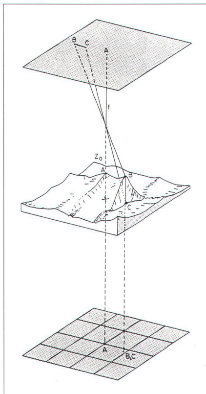
Abb. 5: Verzernte Wiedergabe des Geländes im Luftbild aufgrund seiner zentralperspektivischen Abbildung.
