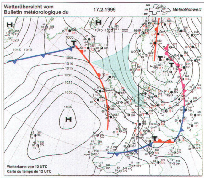
Abb. 1: Druckverteilung vom 17. Februar 1999.
