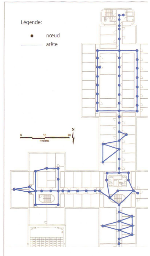
Fig. 1: Extrait du réseau de navigation (nœud/ arête) du campus de l'EPFL.
