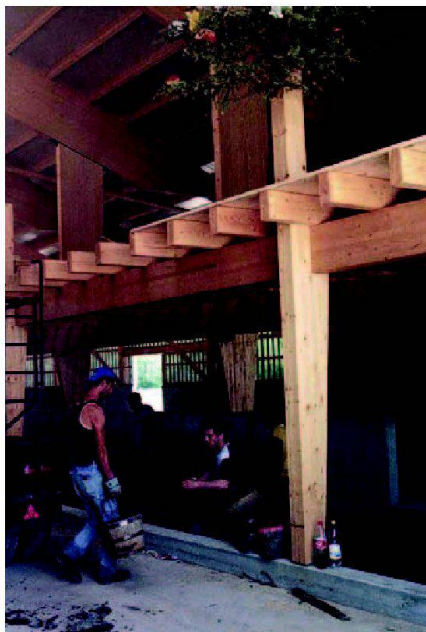
Fig. 3: Maraçon VD: En peu de temps, les éléments préfabriqués en bois sont assemblés sur le chantier. Les finitions intérieures peuvent commencer immédiatement, réduisant d'autant la durée de construction.
