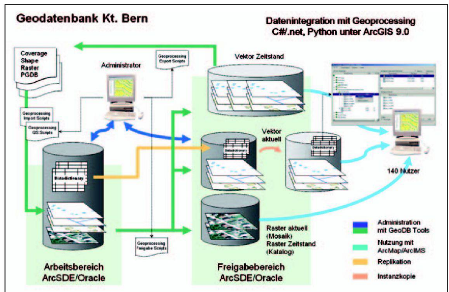
Abb. 1: Hauptprozesse im Geodatenserver Bern.
