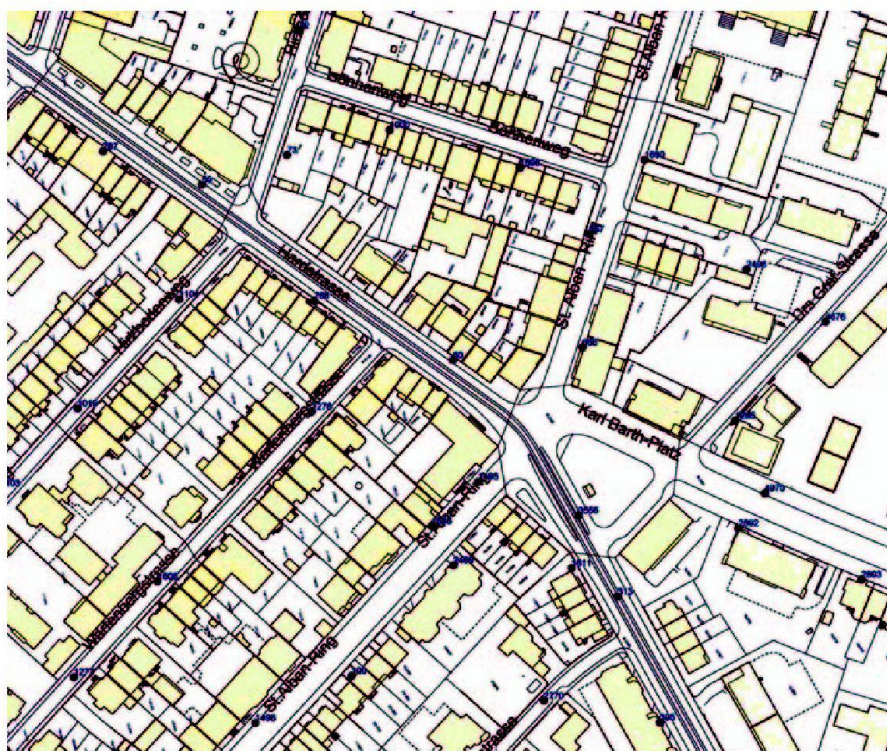
Abb. 4: Hydrantenplan.
