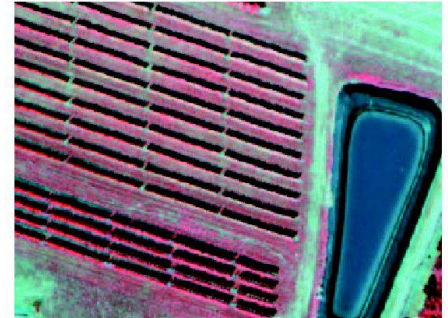
Abb. 3: Ausschnitt des erstellten True Orthophotos als Falschfarbenbild.
