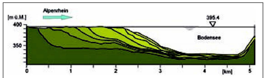
Abb. 2: Längensprofile des Alpenrheindeltas im Bodensee seit 1885 (aus Lambert 1989).
