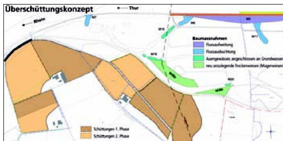
Abb. 2: Überschüttungskonzept.
