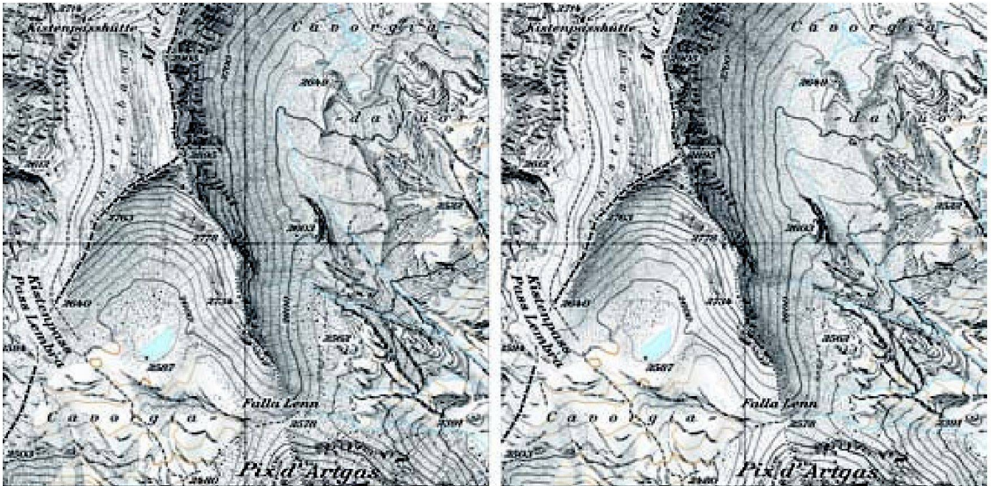
Abb. 5: Manuell erzeugte Gerölldarstellung in der Landeskarte 1:25 000 (links) im Vergleich zur mit ScreePainter automatisch erzeugten Gerölldarstellung und geringfügiger Nachbearbeitung (rechts).
