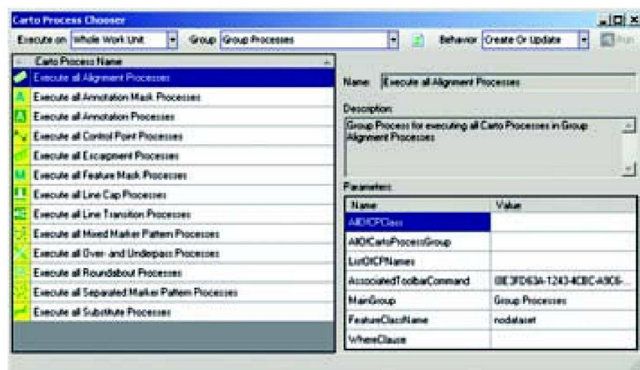
Abb. 4: GUI zum Auslösen von CartoProcesses in der Genius-DB.
