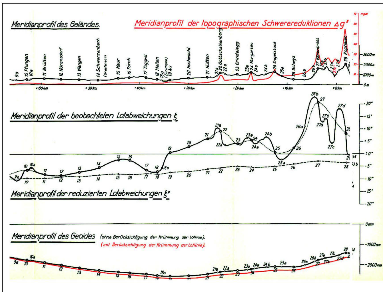
Abb. 4: Astronomisches Profil im Meridian des St. Gotthard (Ausschnitt), Profilbeilage (101 x 30 cm) zu SGK, Band 20, 1939.
