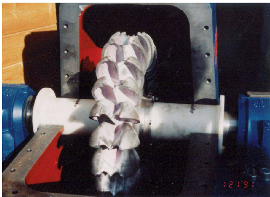
Abb. 9: Peltonturbine Charal.
