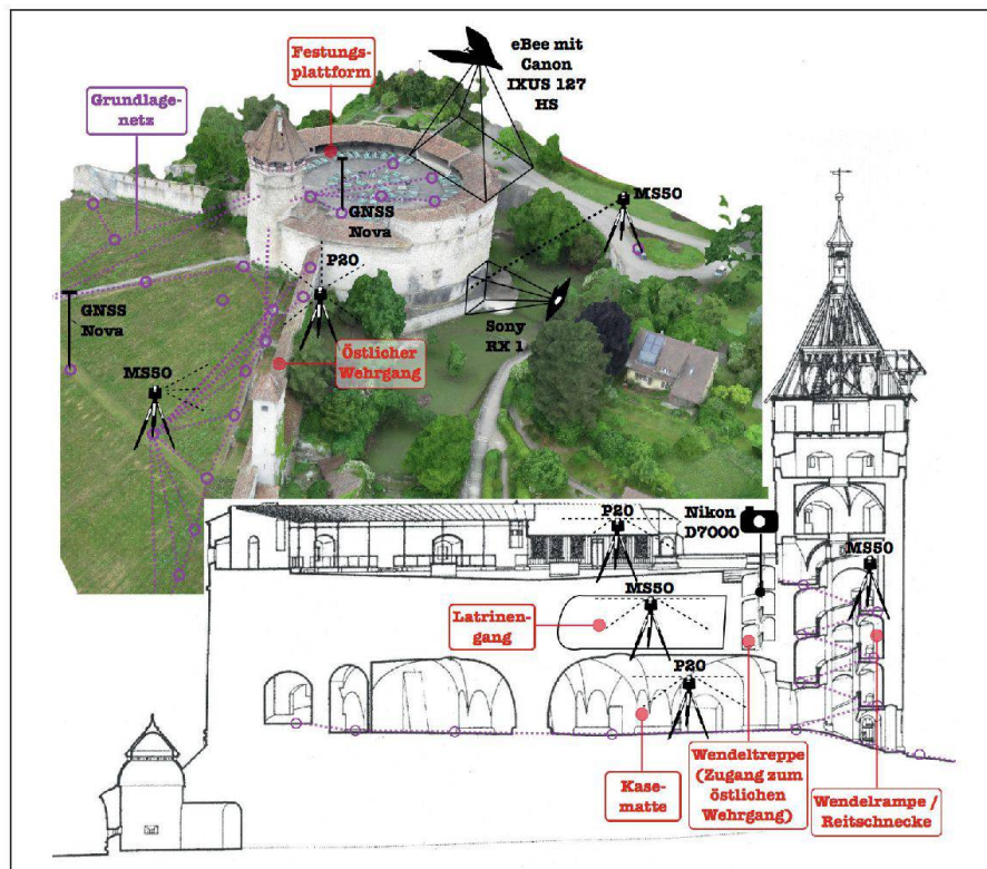
Abb. 1: Übersicht der aufgenommenen Teilobjekte des Munots (rot beschriftet) und der eingesetzten Sensoren. Oben links: Überlagerung auf 3D-Modell aus PhotoScan (oben links); unten rechts: Schnittansicht.
