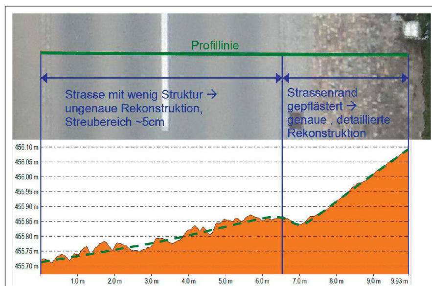
Abb. 2: Beispiel Rekonstruktionsgenauigkeit mittels Dense Image Matching im Strassenbereich, Orthofoto (oben) und Querprofil (unten) – Vergleich Soll-Profil (grün gestrichelt) mit Profil durch rekonstruierte Oberfläche (orange).
