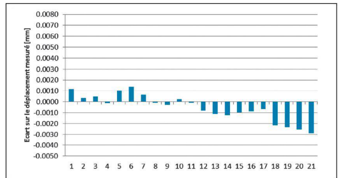
Fig. 1: A gauche, l'expérience constituée par deux blocs de béton sur le banc de l'interféromètre, à droite les écarts mesurés entre l'interféromètre et la corrélation diachronique (1 pixel = 0.1 mm) (M. Prot, 2013).
