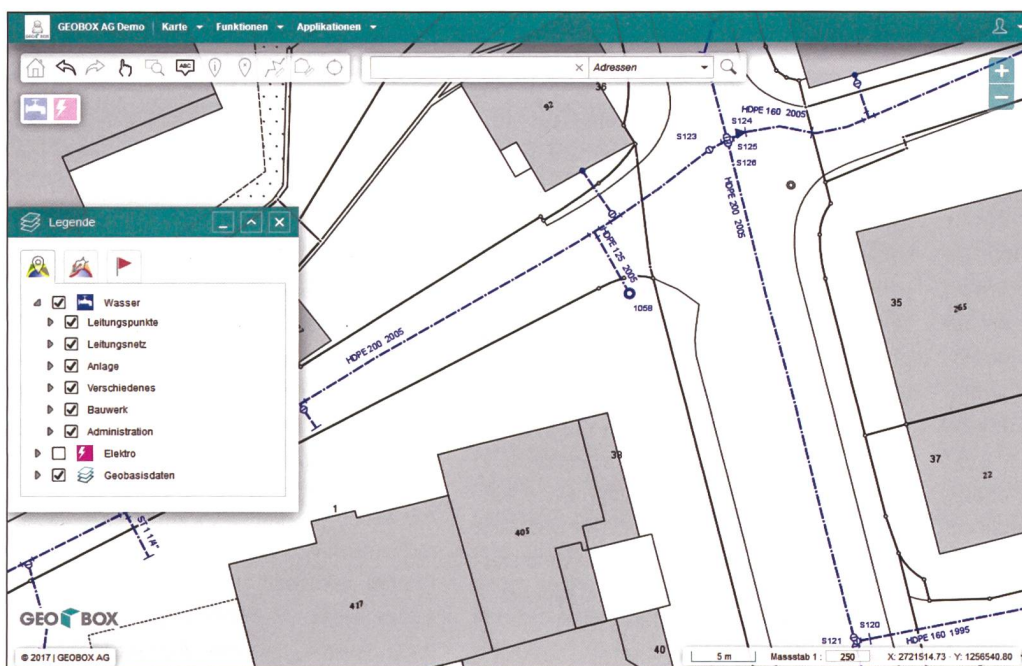
Abb. 1: TBview Kartenansicht.
