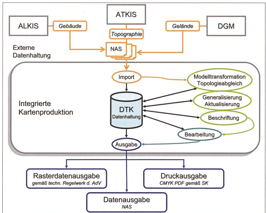
Abb. 1: Integrierte Produktionstechnologieplattform.
