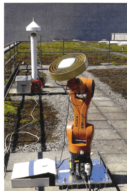
Fig.3: Robot industriel KUKA à six axes sur le toit de l'Institut de géodésie et de photogrammétrie de l'ETH Zurich au Höggerberg. L'antenne de référence est visible à l'arrière-plan.
