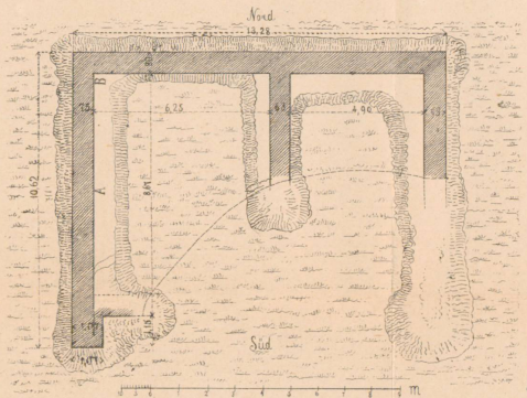
F 2 Grundriss (200)
