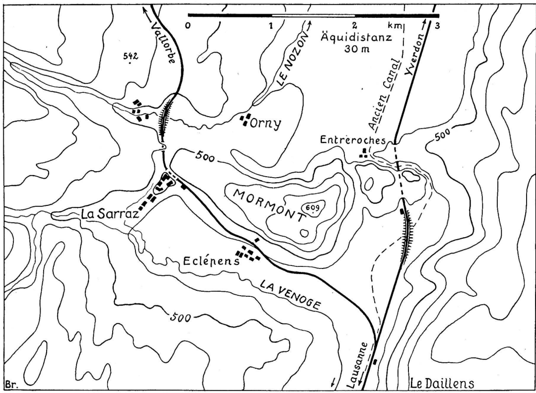
Bild 19. Sporn-Spizentunnel bei La Sarraz und Entreröches an der europäischen Hauptwasserscheide. (Nach der Siegfriedkarte.)
