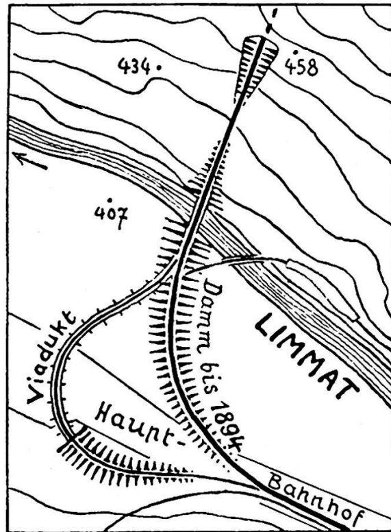
Bild 2. Steigungsdam (Form B b), 1894 durch einen Steigungsviadukt ersetzt, auf der Strecke Zürich-Oerlikon. (Nach der Siegfriedkarte.)
