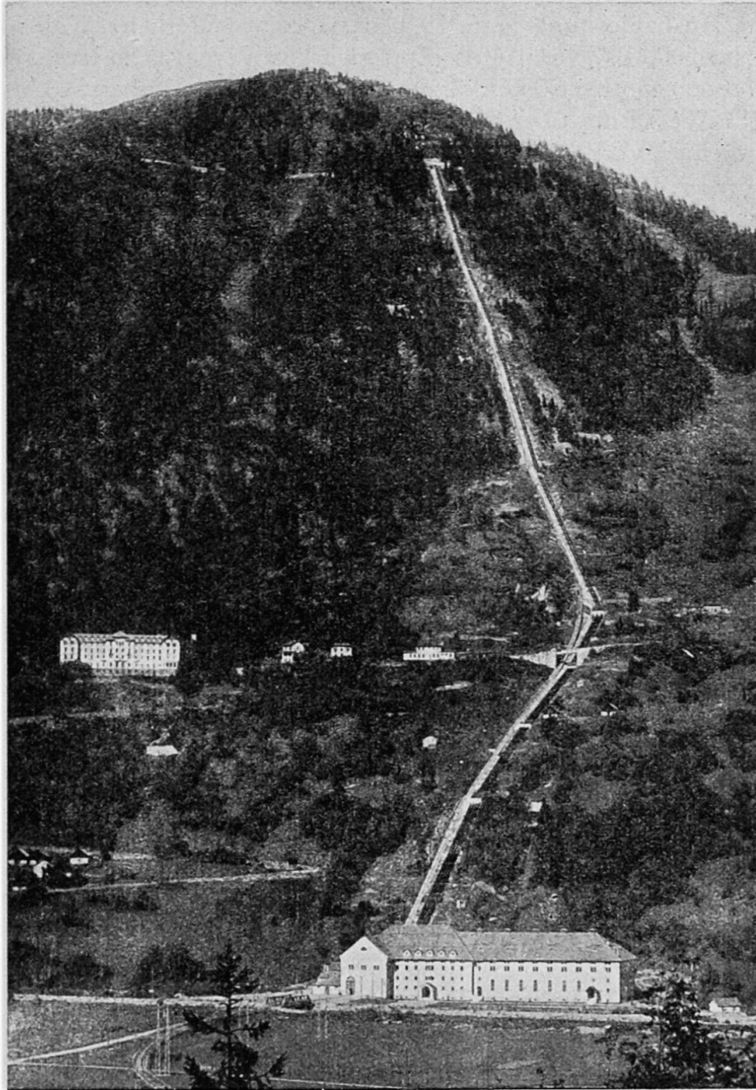
Abb. 8. Ritomwerk im oberen Tessental als Typus eines größeren Hochdruckwerkes (maximale Spitzenleistung: 41000 kW). In 4 Druckleitungen wird das Wasser mit einem mittleren Gefälle von 824 m zur Zentrale geleitet. Klischee vom Eidg. Amt für Wasserwirtschaft.
