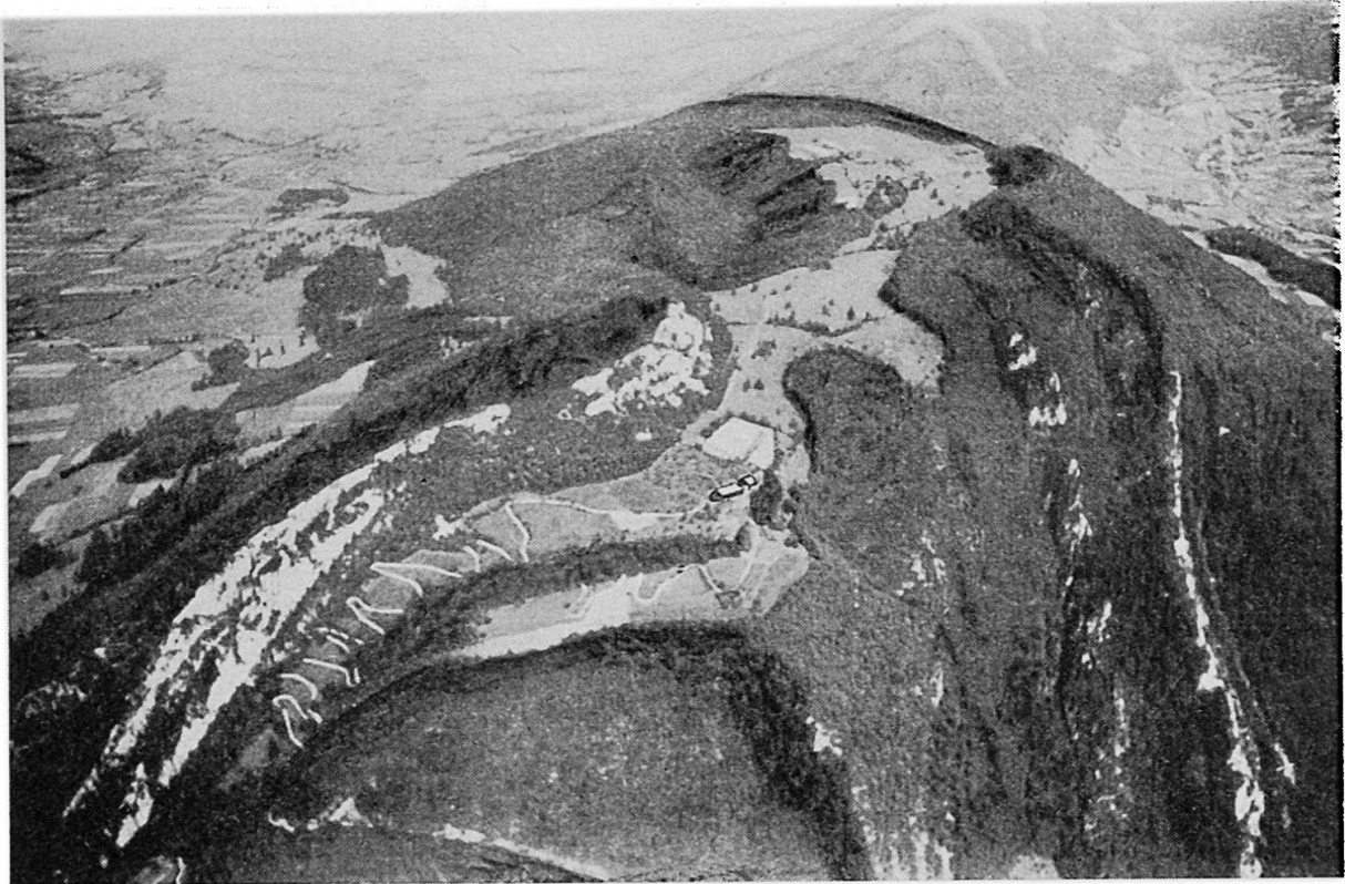
Fig. 65: Aufgebrochenes Faltengebölbe im Kettenjura. (Südlich Bassecourt, vgl. auch Anaglyphentafel 12.) Durch die Erosion wurde eine weichere Schicht im Kern der Antiklinalen bloßgelegt, wodurch eine konkave Geländeform erzeugt wurde (Anfangsentwicklung eines Antiklinaltales). Im Antiklinaltal unserer Abbildung liegt eine Familienwirtschaft, natürlich begrenzt durch die ausstreichenden harten, mit Wald bedeckten Kalkschichten. Der Zufahrtsweg (kurvenreiche Straße links im Bild) benützt ebenfalls die weiche Schicht. Verschiedene Landnutzungszonen sind durch Grünhecken voneinander getrennt. Im Vordergrund ist die Ostseite der Klus S Bassecourt sichtbar. (Flugaufnahme von T. Hagen, behördlich bewilligt am 29. August 1950.)
