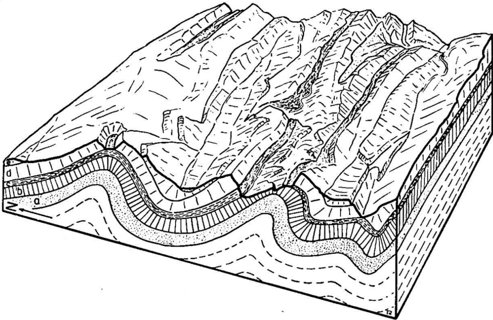
Fig. 73: Geologisches Blockdiagramm.
