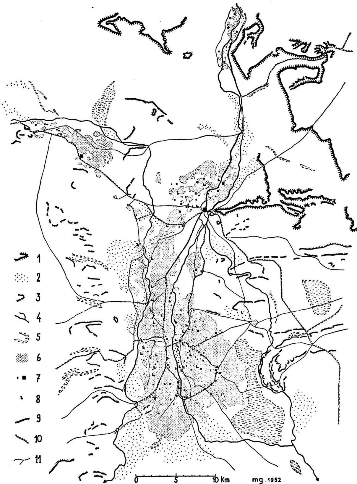
Abb. 6 Oase Tafilalet: Boden und Siedlung. 1 Kreb, 2 zusammenhängende Dünengebiete, 3 Felsköpfe und Schichtrippen, 4 Oued Rheris und Ziz, 5 Sebkhha oder versalzte Böden, 6 Oasengebiet, 7 bewohnte Siedlungen, annähernd flächentreu, 8 Ruinen von Siedlungen, 9 Straße, 10 Pisten (fahrbar), 11 Wege. (Grundlage Karte 1:100 000)
