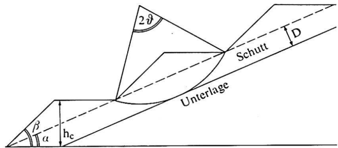
Fig. 7 Geometrie eines Schutthanges.
