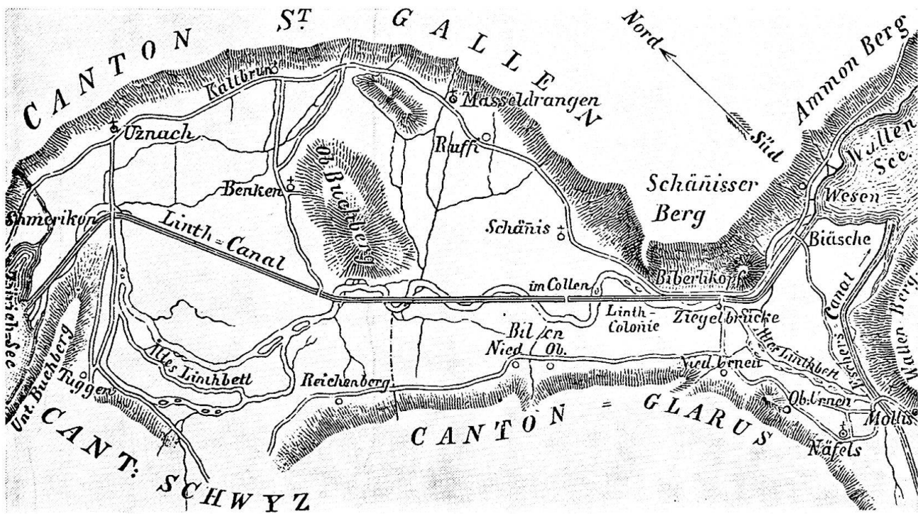
Abb. 2 Der alte Linthlauf und das unter der Leitung Eschers durchgeführte Korrektionswerk.
