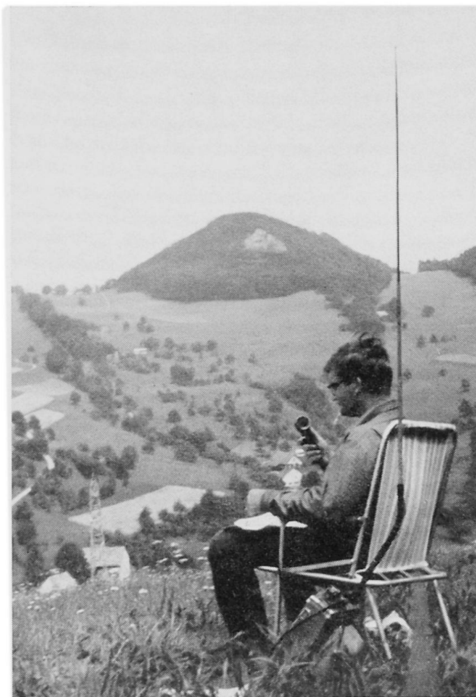
Abb. 3 Der Mitarbeiter an der P-S übersieht das Gelände. Von seinem festen Standort aus leitet er die Kartierung über den Funk (SE-101, Monophonbetrieb) und fixiert fortlaufend die Angaben der G-S auf dem Plan.
