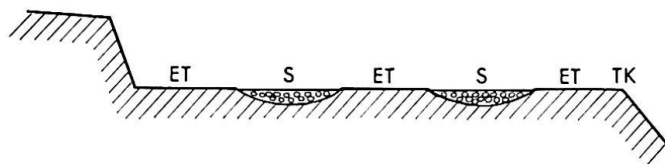
ET Erosionsterrassenfläche S Sekundärschotter als Rinnenfüllung TK Terrassenkante
