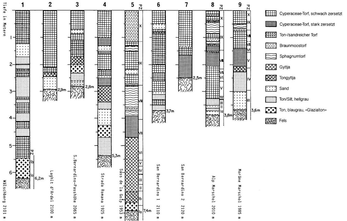
31 Abb. 3 Bohrprofile der Verlandungs-Niedermoore am Bernardin-Paß
