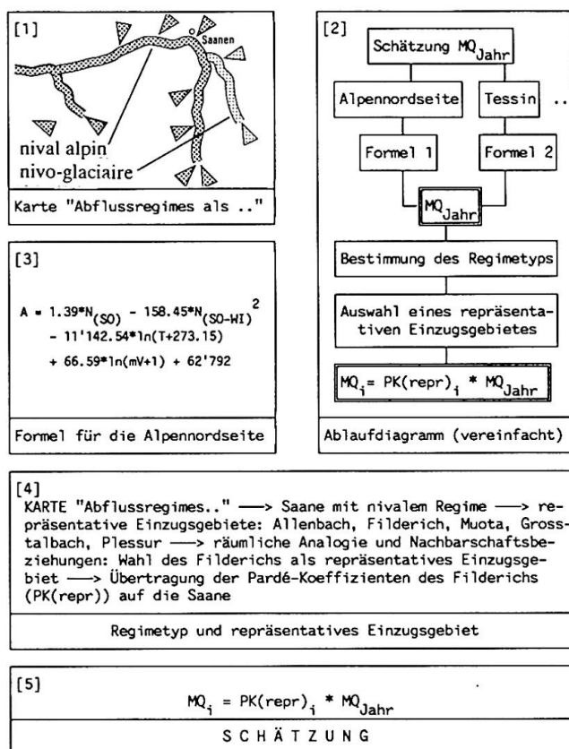
Fig. 3 Zur Abschätzung von langjährigen mittleren Monatsabflüssen mit Hilfe der Tafel «Abflußregimes» des «Hydrologischen Atlas der Schweiz» – Beispiel: Saane in Saanen; Abkürzungen: N_{(SO)} : Gebietsniederschlag im Sommerhalbjahr [mm]; N_{(SO-WI)} : Verhältnis Sommer- zu Wintergebietsniederschlag; T: mittlere Jahrestemperatur [°C]; mV: mittlere areale Vergletscherung [%]
