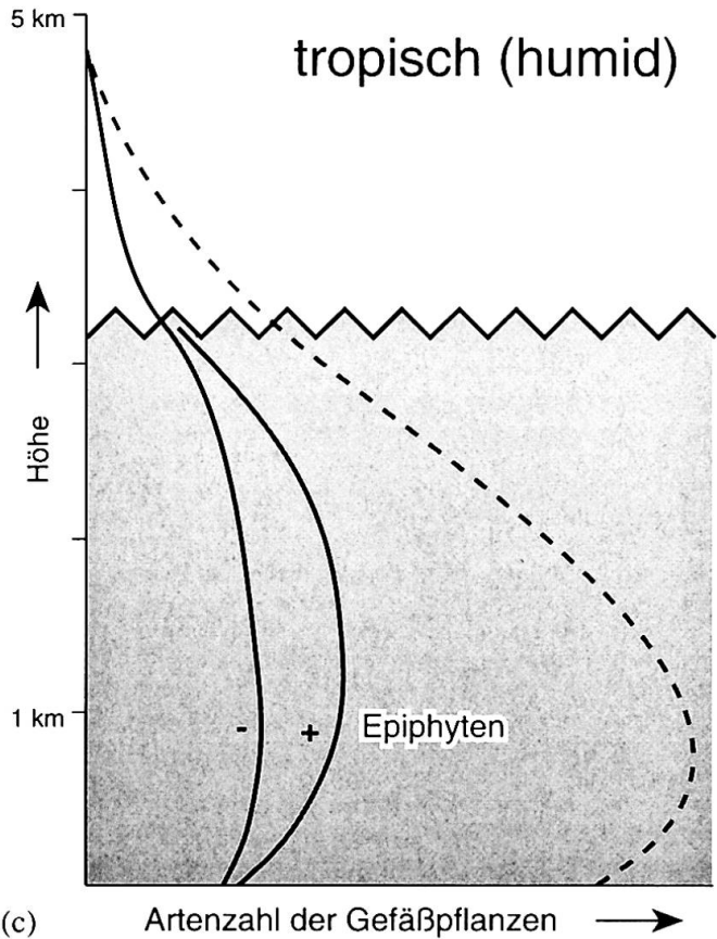
Abb. 2: Höhenwandel der Artenvielfalt pro gleich großen Flächen ( \beta -turnover) in natürlichen Beständen, die der jeweiligen klimatisch induzierten Vegetation eines Höhenniveaus entsprechen; modellhaft dargestellt für Gebirge verschiedener Klimazonen Lapse rates of species-richness per plot of the same size ( \beta -turnover) in natural stands, demonstrated as models for mountains of different zones of climate Courbes d'altitude de la diversité d'espèces ( \beta -turnover) sur parcelles de la même superficie en populations naturelles, présentées de manière exemplaire pour des massifs de différentes zones climatiques
