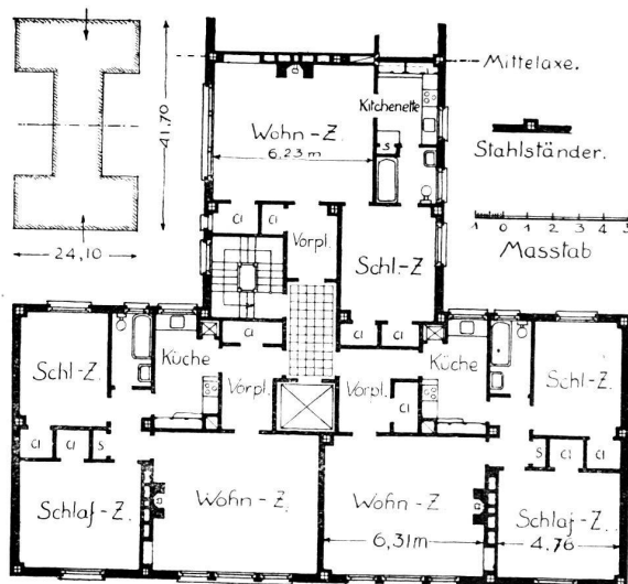
Fig. 1. Plan d'une maison locative à New-York, 12 étages. A chaque étage, 6 appartements de 2 à 3 pièces (cuisine non comprise). Construction en acier avec parois en briques. A gauche en haut, plan du bâtiment complet — cl. - closet, c'est à dire armoire profonde, sorte de penderie. Wohnz. - chambre commune, Schlafzimmer - chambre de coucher, Vörpl. - Vestibule.
