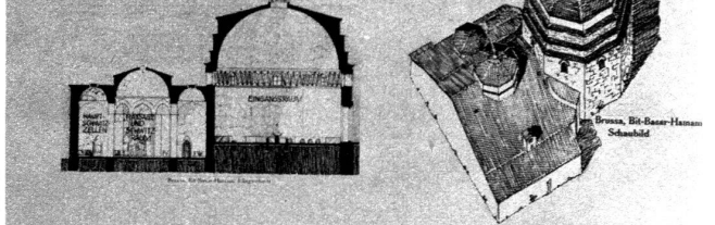
Vue extérieure des coupoles d'un haman. Plan, coupe et vue axonométrique du haman Bit-basar à Brousse.
