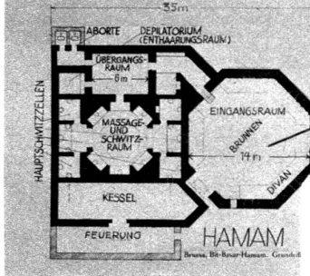
Vestibule d'entrée avec fontaine et divan, étuve et salle à massage, dégagement, lieux d'aisance, dépilatoire, cellules de sudation, chaudière, chauffeerie.
